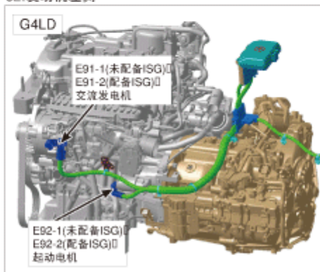
32. 发动机左侧
