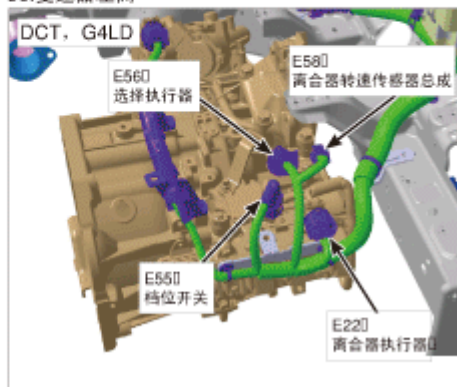
36. 变速器左侧
