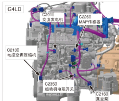
33. 发动机左侧
