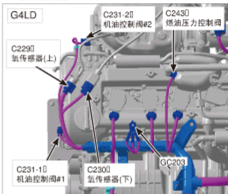
31. 发动机顶部
