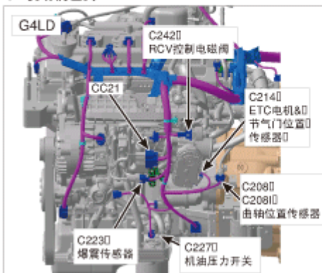
34. 发动机左侧
