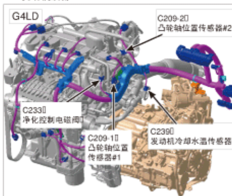
35. 发动机后部
